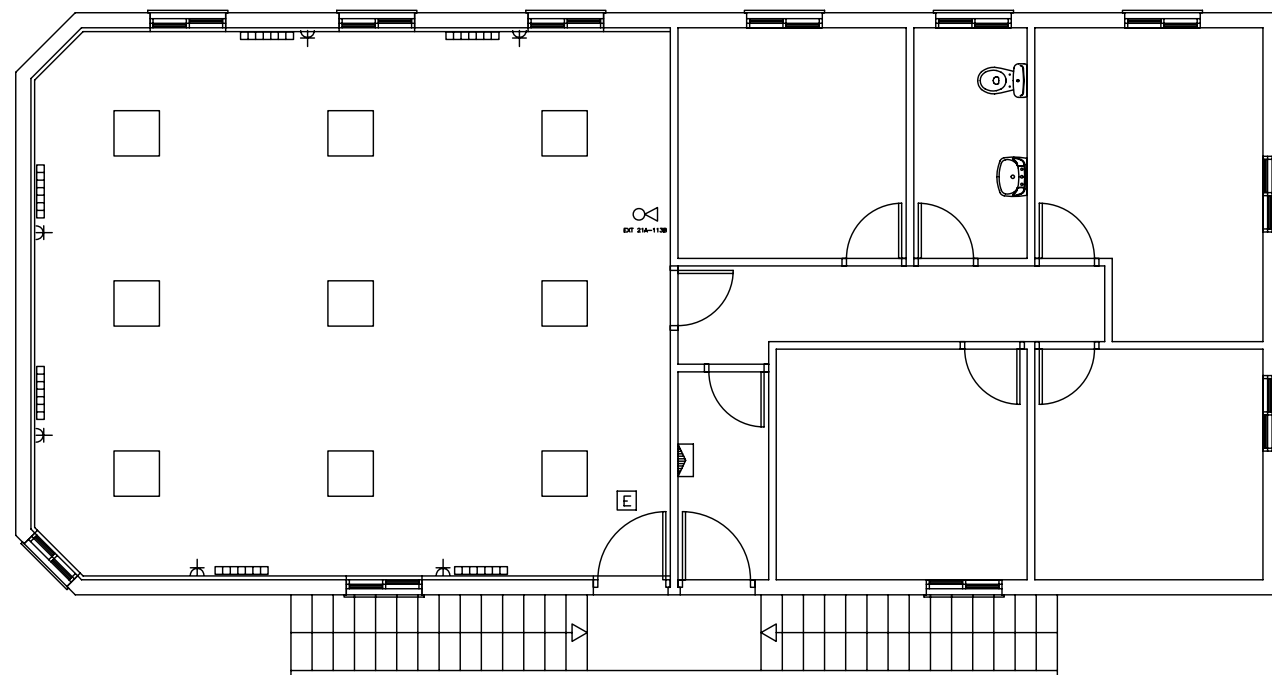
PLANTA PRIMERA (ELECTRICIDAD)
