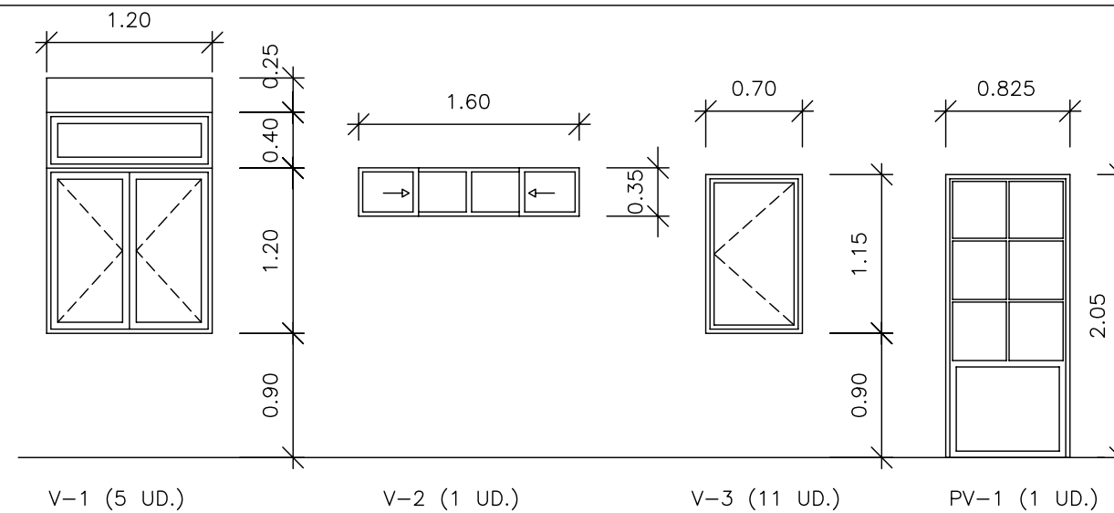
ESQUEMAS DE CARPINTERIA
