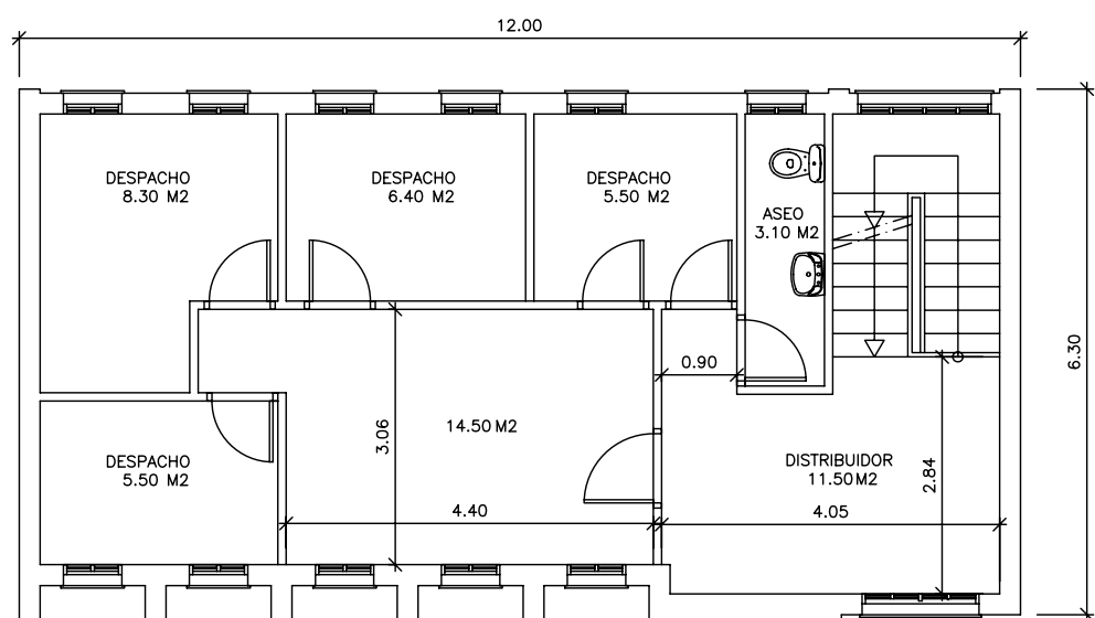
PLANTA PRIMERA
