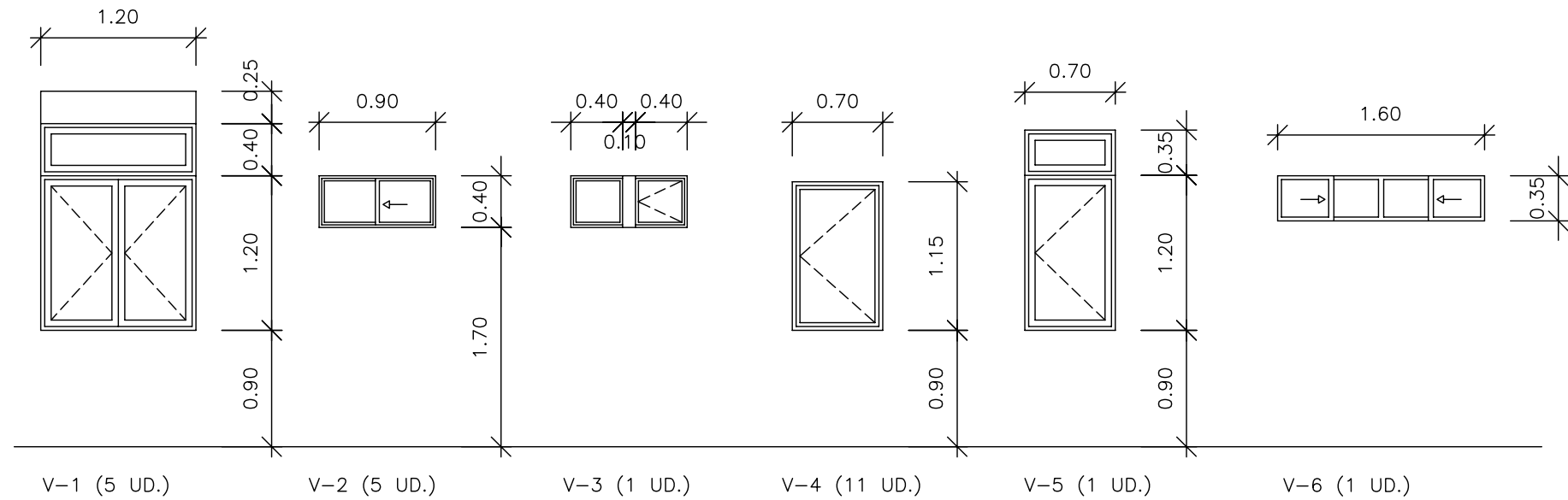
ESQUEMAS DE CARPINTERIA
