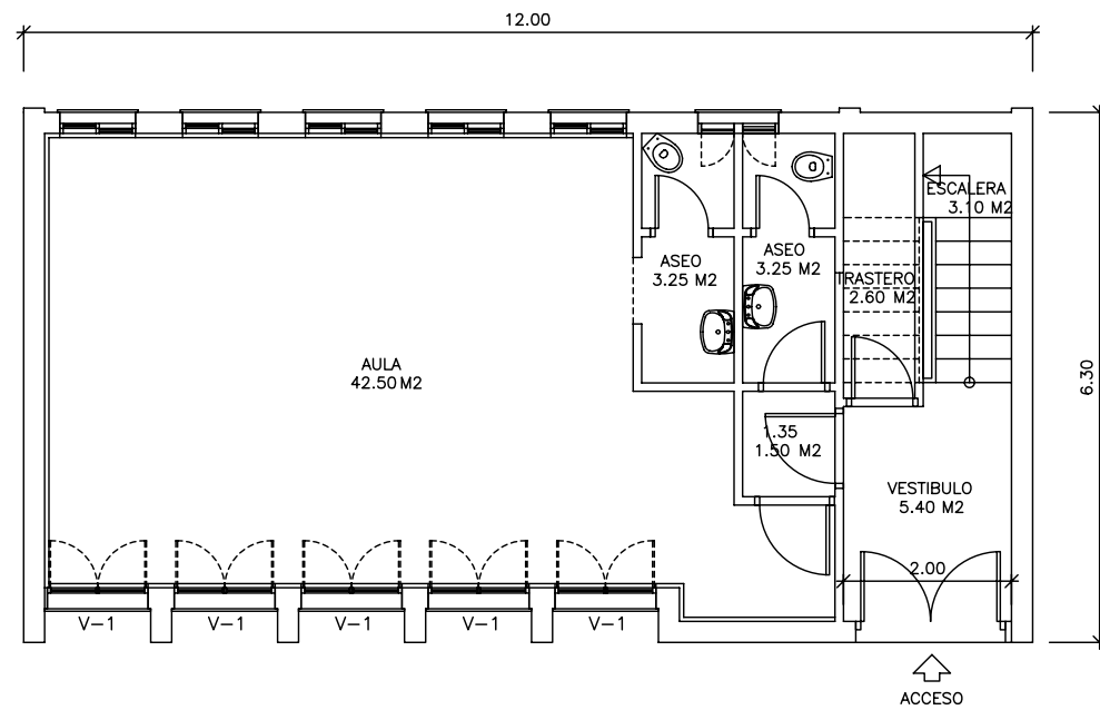
PLANTA BAJA
