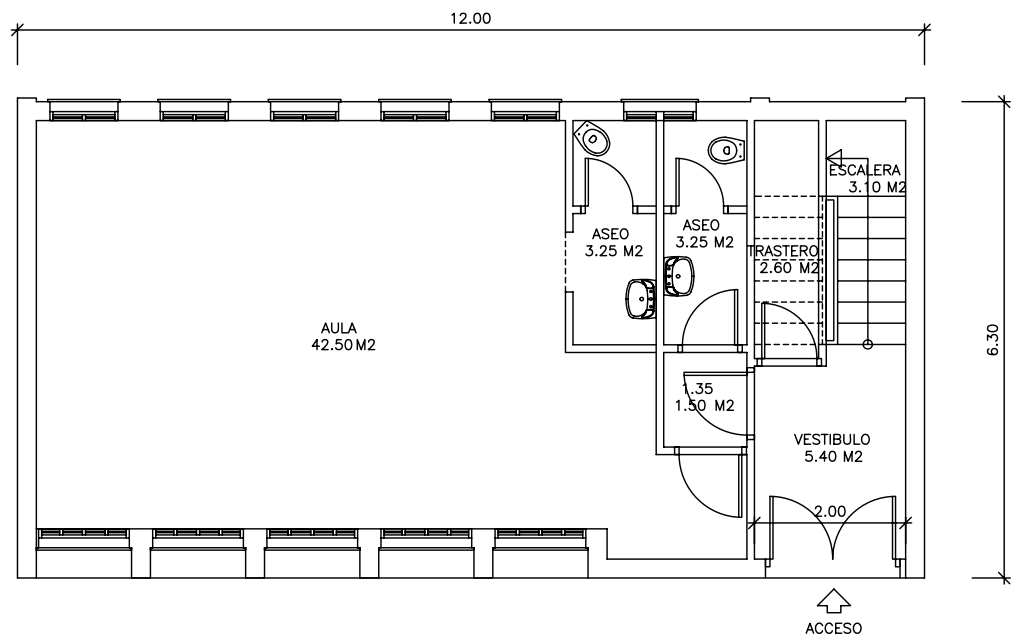
PLANTA BAJA
