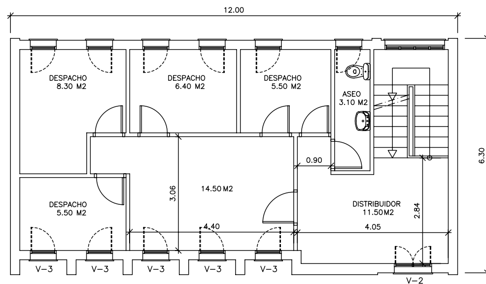
PLANTA PRIMERA
