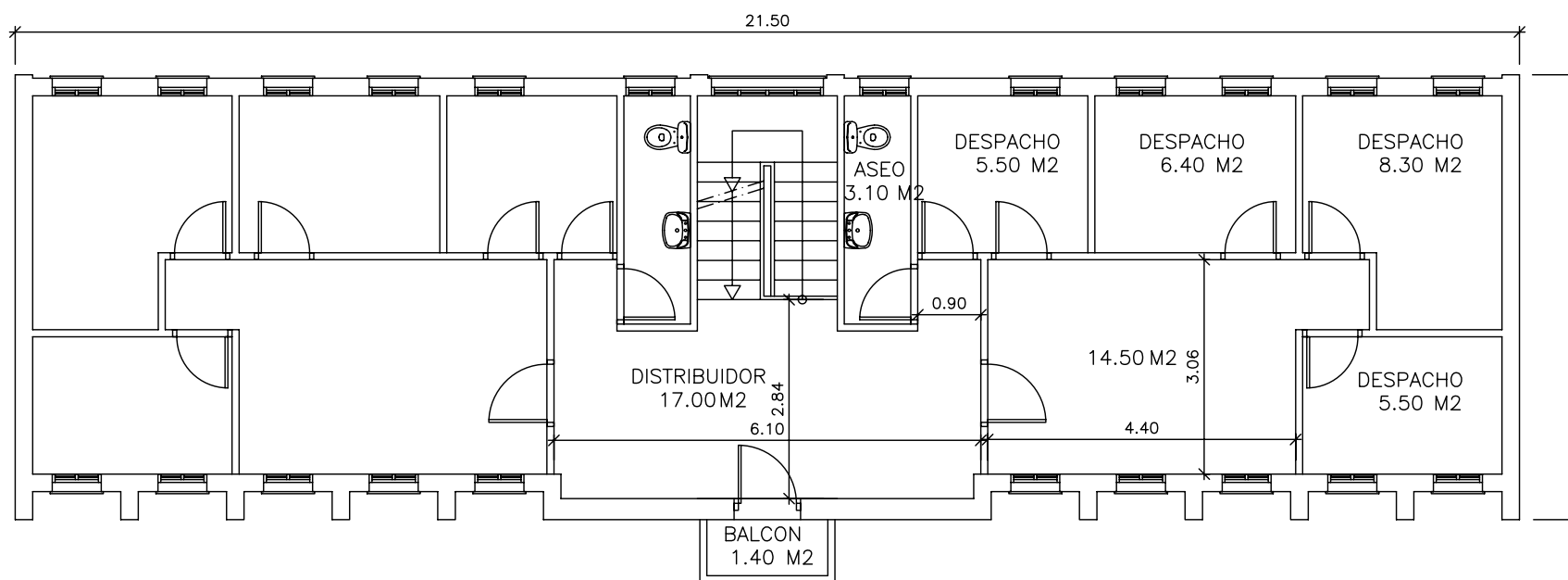
PLANTA PRIMERA
