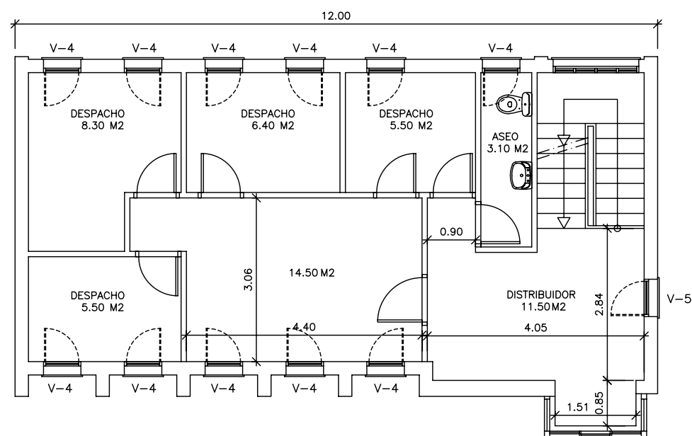
PLANTA PRIMERA
