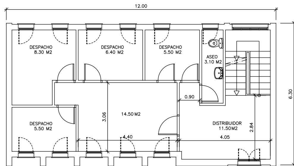
PLANTA PRIMERA
