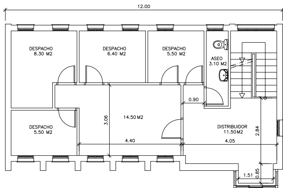
PLANTA PRIMERA
