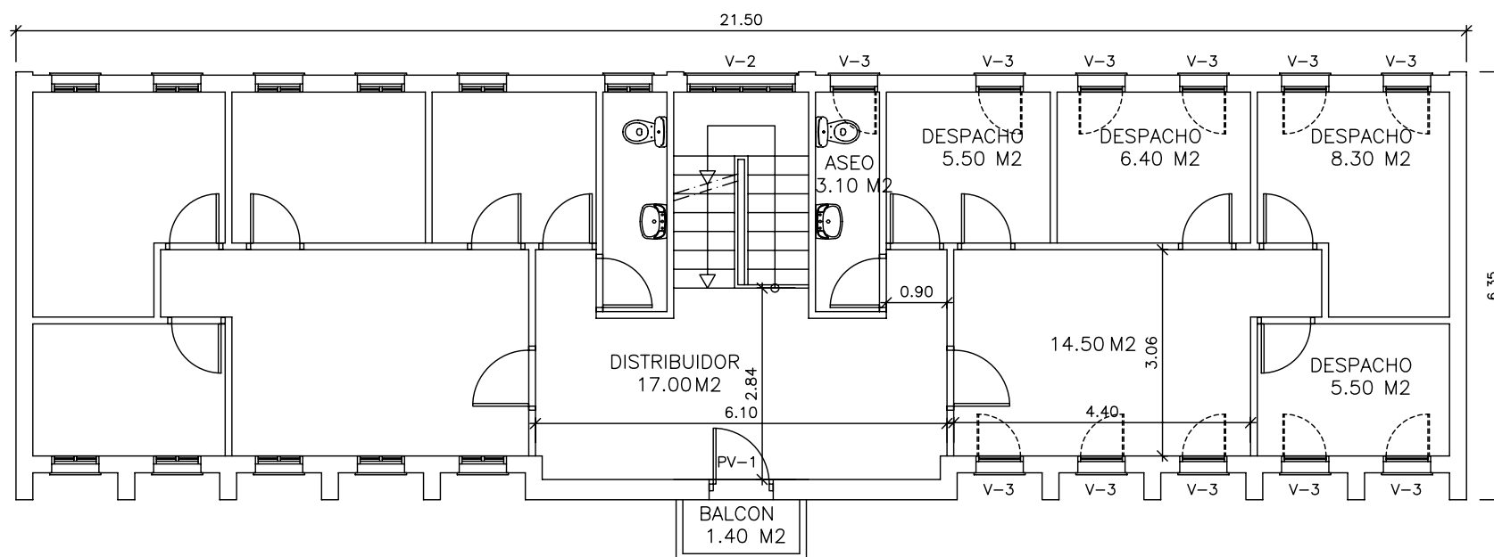
PLANTA PRIMERA
