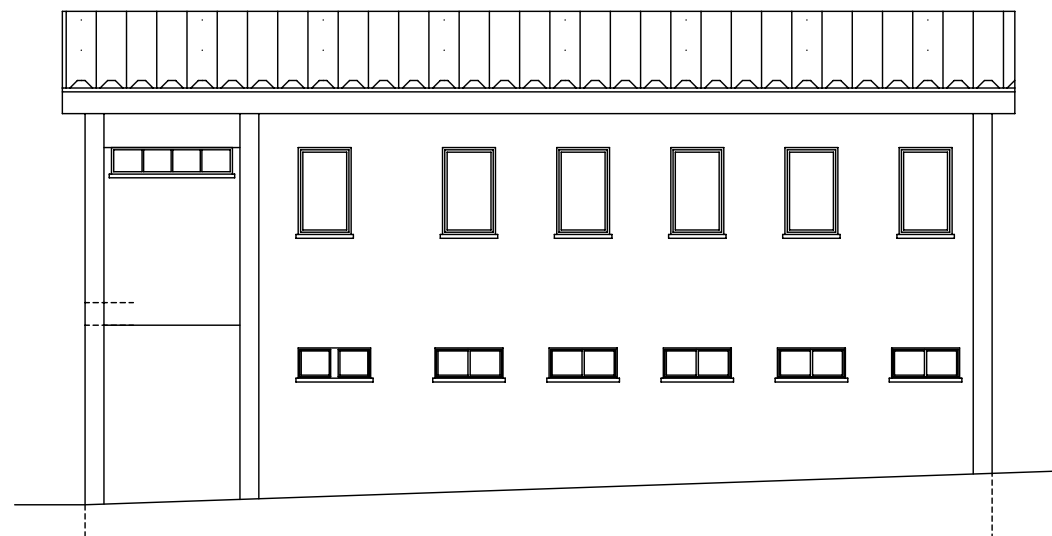
ALZADO POSTERIOR
